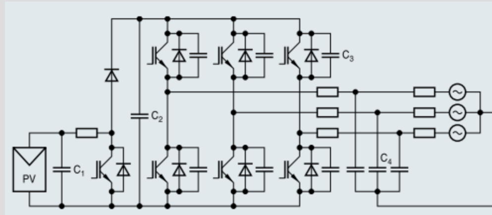
Epcos MKP FC Solar Inverters
