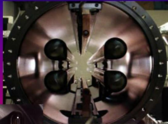
CESR separator
